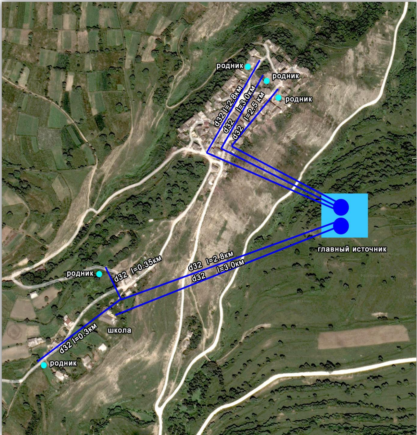
Схема водопроводных сетей в селе Канасираги
