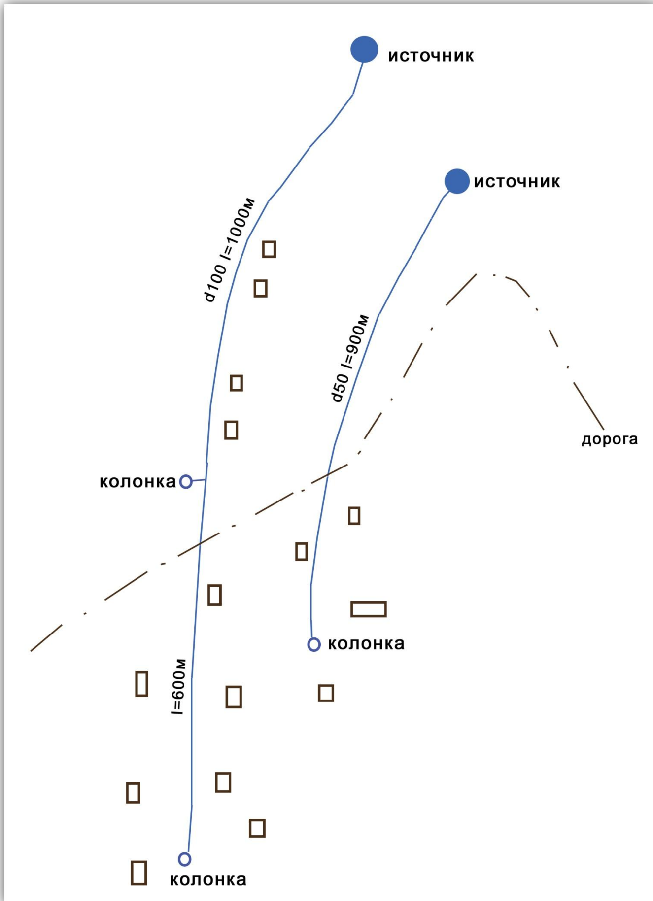
Схема водопроводных сетей в селе Балтамахи
